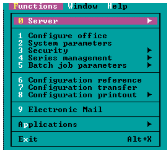
Fig 9.1 MODSYSCF : Functions
